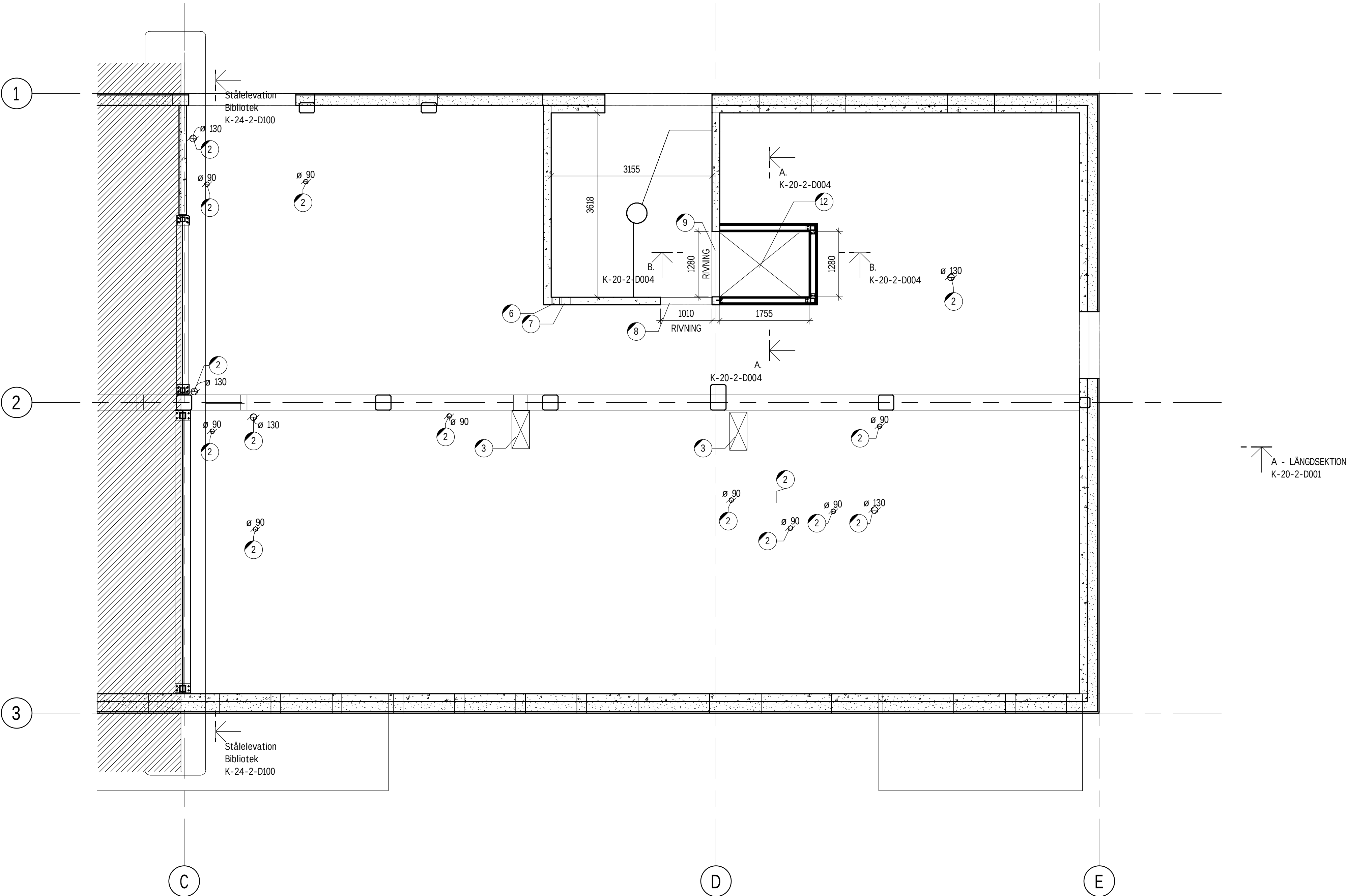
PLAN 1 - Del 2 1 : 50
